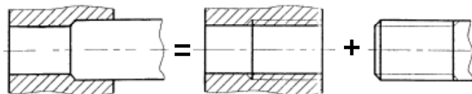
Assemblage Tige filetée/Trou taraudé (ou Vis/Ecrou)
